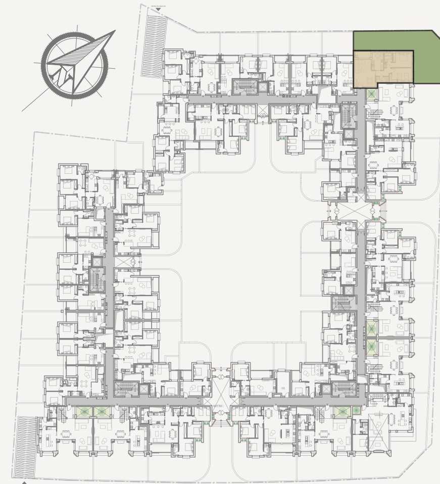
APPARTEMENT D-0.5
